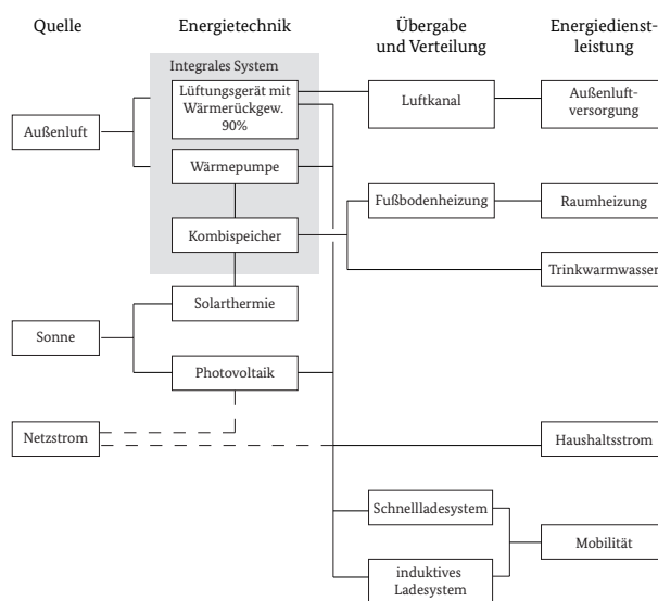
Abb. 14: Beispielhafte Darstellung eines vorab definierten Energieversorgungskonzeptes
