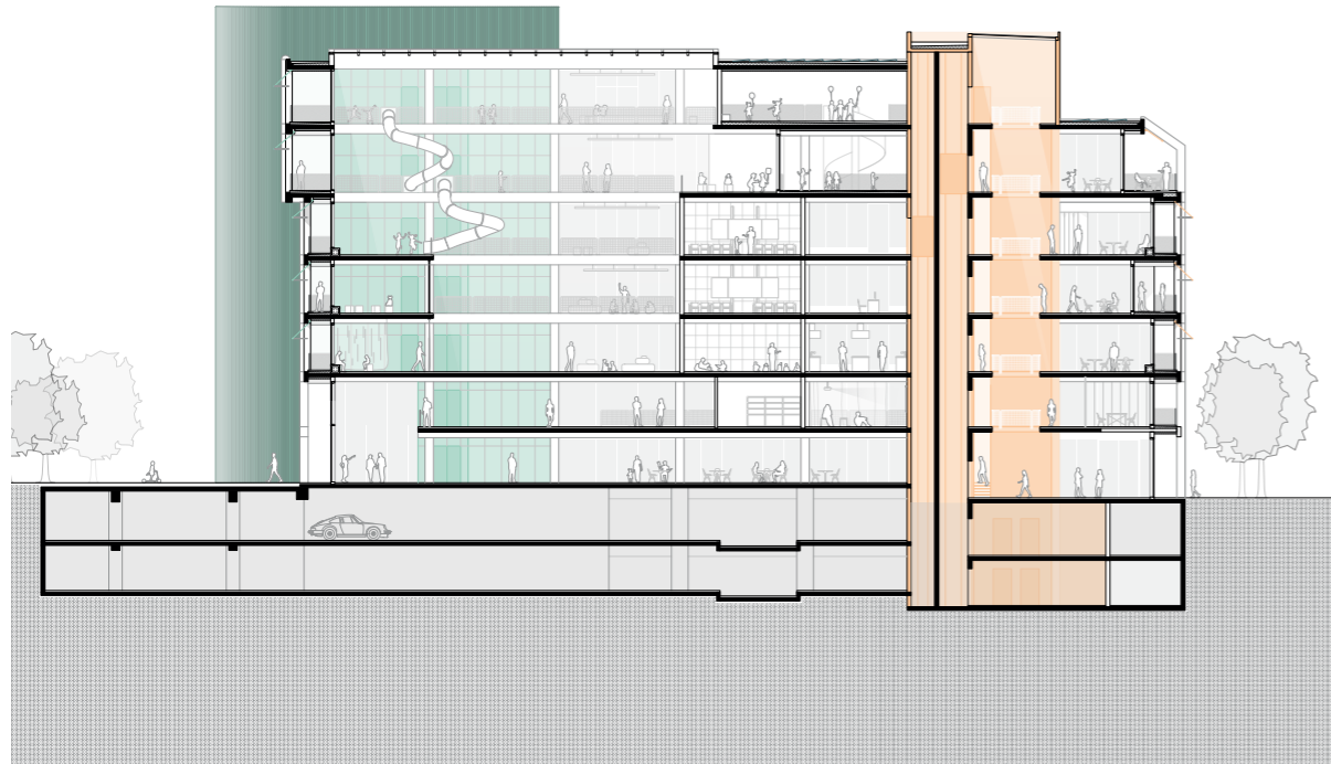
Schnitt A-A
