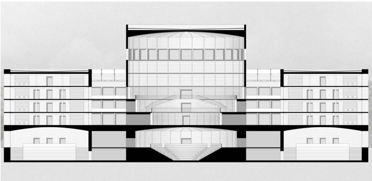
Schnitt AA
