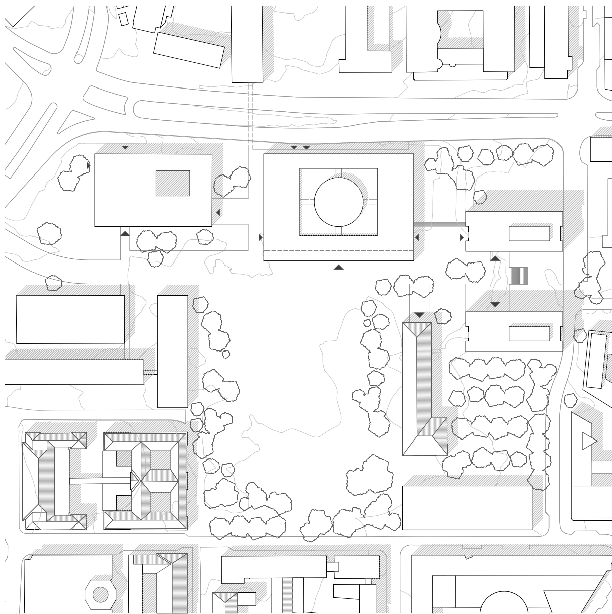
Lageplan
