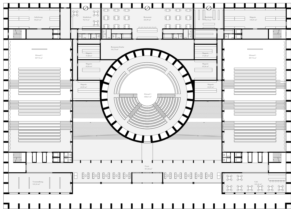
Erdgeschoss Plan
