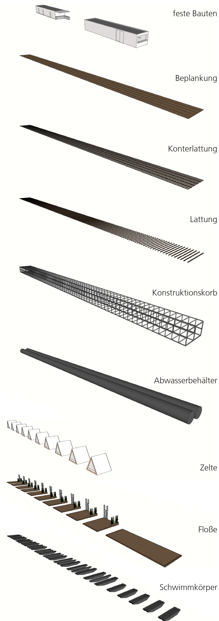
Explosionszeichnung
