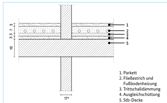
Abb. 1: Herkömmliche Bauweise – Massivbau Geschossdecke
