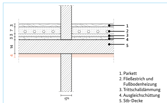
Abb. 2: Abweichende Bauweise – Massivbau Geschossdecke
