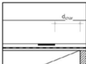
Abbildung 28: Außenwand-Deckenanschlüsse Holztafelbau / Massivholzbau mit Spaltmaß s \leq 2,0 mm
