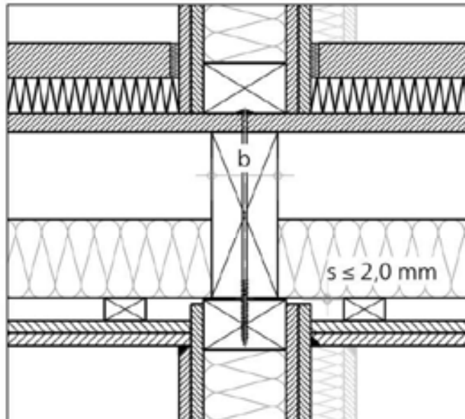
Abbildung 8: Trennwand-Deckenanschlüsse Holztafelbau mit Spaltmaß s \leq 2,0 mm
