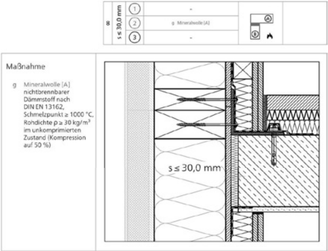
Abbildung 36: Holztafelbau für nichttragende Außenwand / mineralischer Massivbau mit Spaltmaß s \leq 30,0 \text{ mm}
