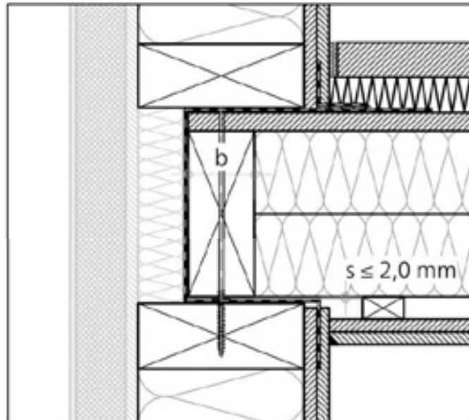
Abbildung 7: Außenwand-Deckenanschlüsse Holztafelbau mit Spaltmaß s \leq 2,0 mm
