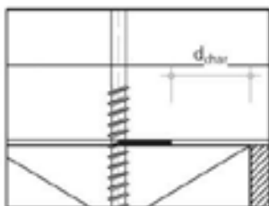
Abbildung 30: Trennwand-Deckenanschlüsse Holztafelbau / Massivholzbau mit Spaltmaß s \leq 2,0 mm
