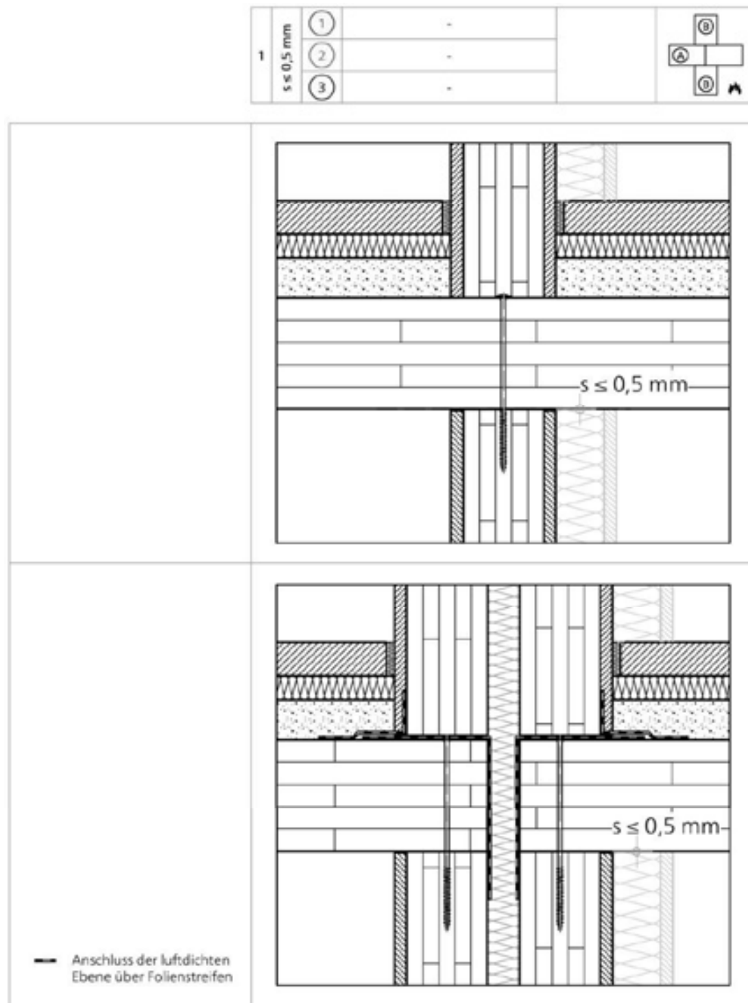
Abbildung 14: Trennwand-Deckenanschlüsse Massivholzbau mit Spaltmaß s \leq 0,5 \text{ mm}
