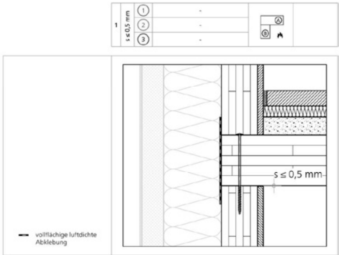
Abbildung 13: Außenwand-Deckenanschluss Massivholzbau mit Spaltmaß s \leq 0,5 \text{ mm}
