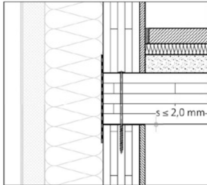
Abbildung 15: Außenwand-Deckenanschlüsse Massivholzbau mit Spaltmaß s \leq 2,0 mm
