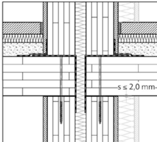
Abbildung 17: Trennwand-Deckenanschlüsse Massivholzbau mit Spaltmaß s \leq 2,0 mm
