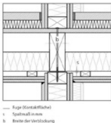
Abbildung 1: Definition von Fuge und Spaltmaß s
