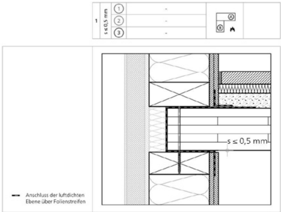
Abbildung 26: Außenwand-Deckenanschluss Holztafelbau / Massivholzbau mit Spaltmaß s \leq 0,5 \text{ mm}
