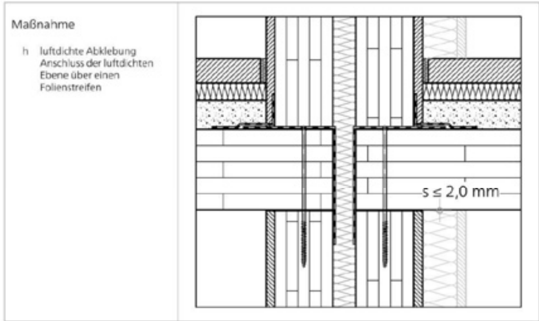
Abbildung 19: Trennwand-Deckenanschluss Massivholzbau mit Spaltmaß s \leq 2,0 mm
